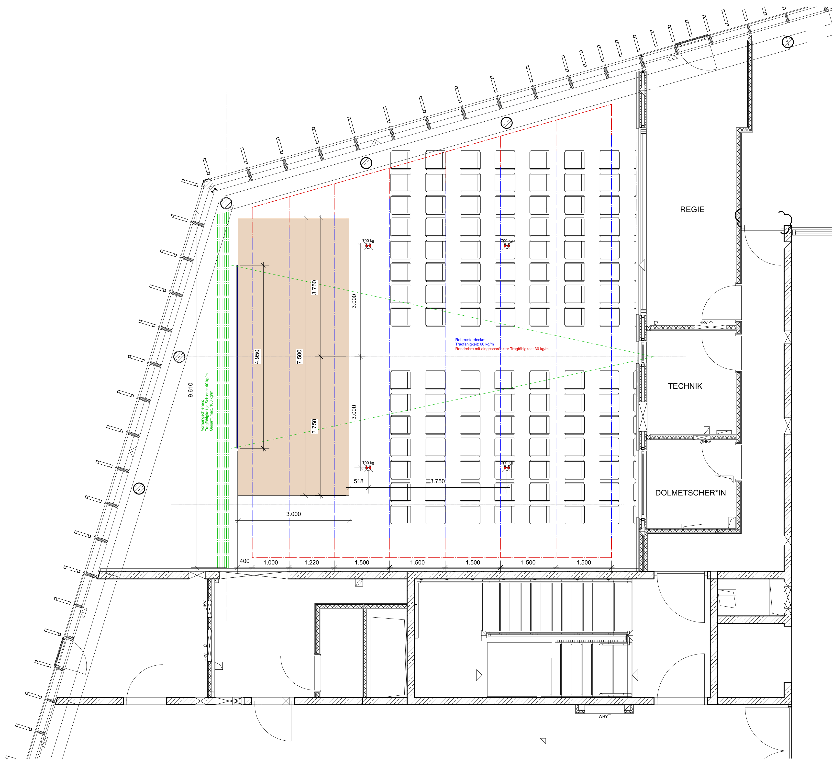
GR OG2 1:50
